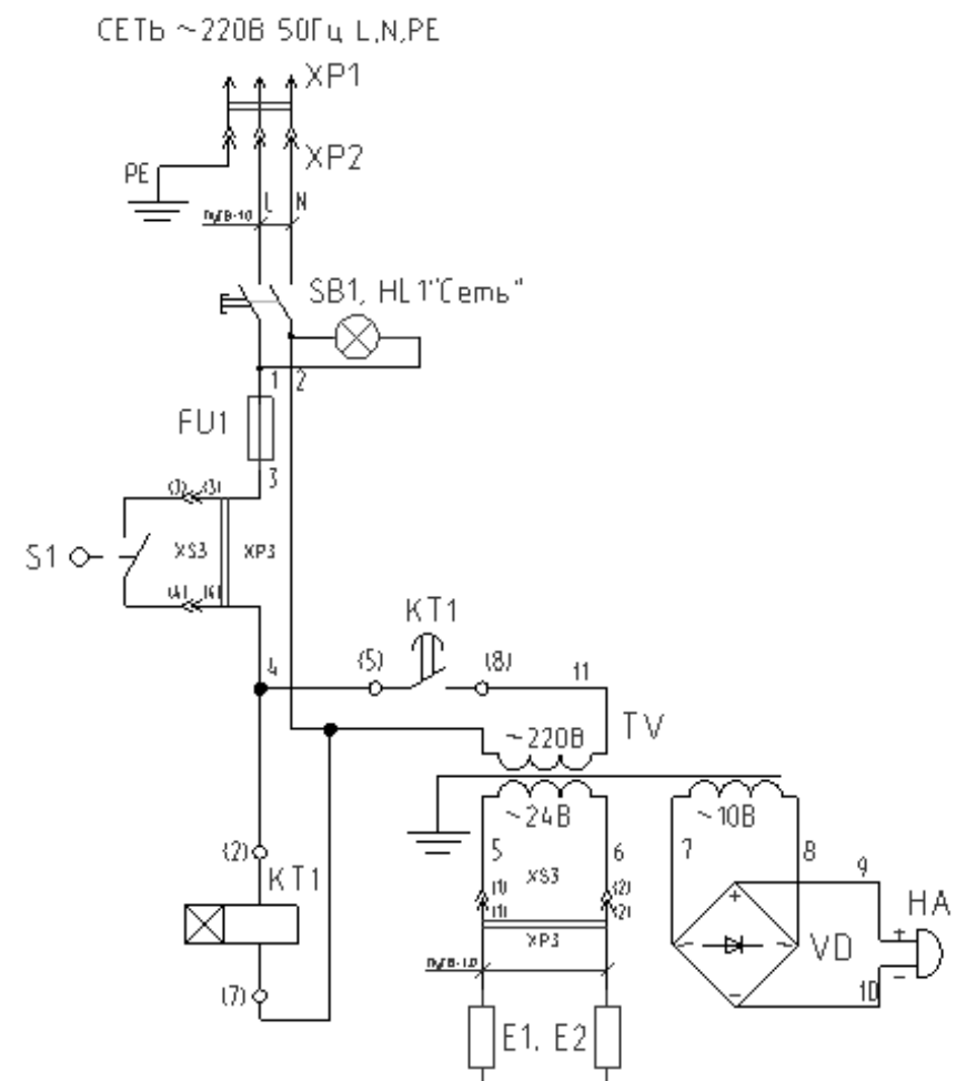
Рисунок 3. Электрическая схема
