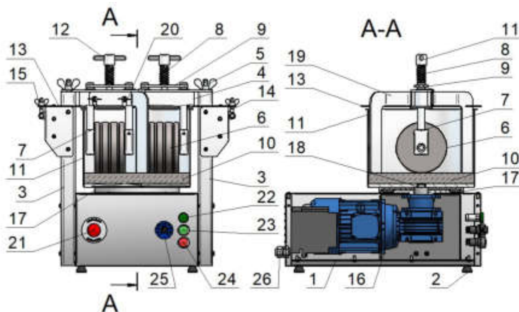
Рис. 2 Устройство меланжера
