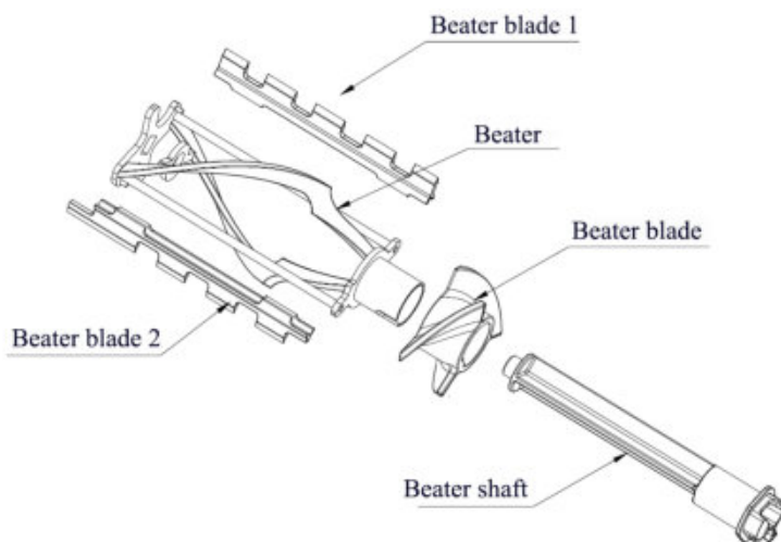
Сборка миксера
